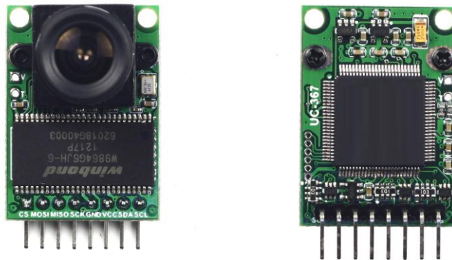
Figure 1 ArduCAM Mini 5MP Plus
